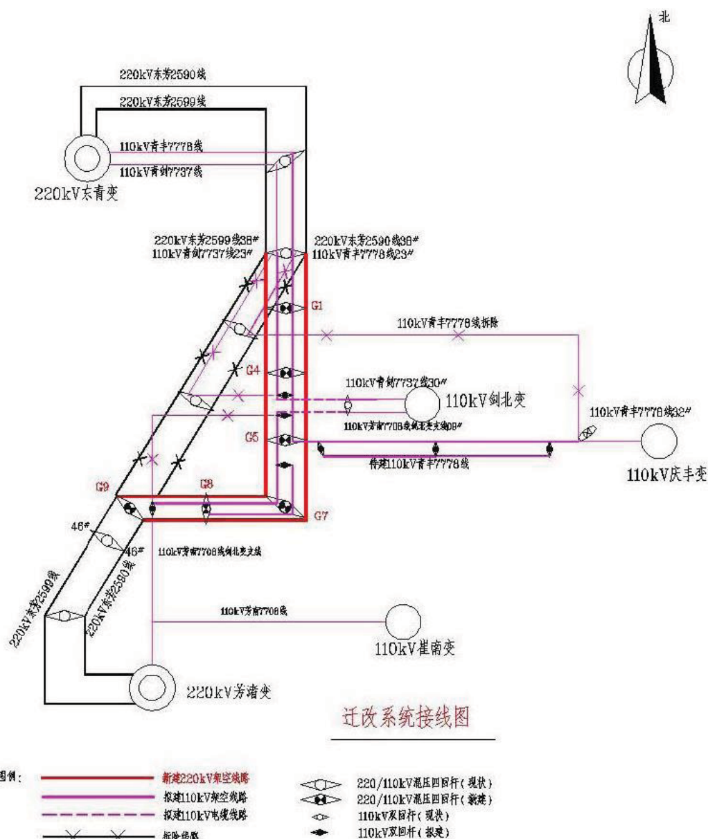
图 2-2 220kV 东芳 2590/2599 线 (38#-46#) 接入系统方案图
